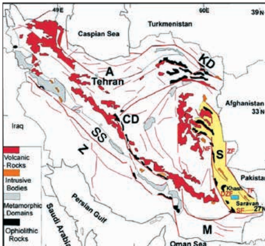
شکل ۱- گستره مورد بررسی در نقشه پهنه‌بندی ساختاری ایران با مستطیل آبی رنگ در پهنه سیستم (بخش زرد رنگ) و جنوب شهر خاش نشان داده شده است. M: مکران، Z: زاگرس، SS: سندج- سیرجان، A: البرز، KD: کپه داغ، CD: ایران مرکزی، TF: گسل تلخ آب، DZF: گسل دامن- زابلی، SF: گسل سرتنگ، NF: گسل نه باختری و ZF: گسل زاهدان.
