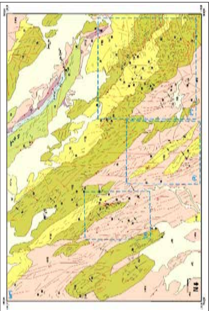
شکل ۲- الف) نقشه زمین شناسی گستره مورد بررسی (موسوی، ۱۳۸۴)، محدوده‌های ب، ج و د با بزرگنمایی بیشتر در شکل های بعدی نشان داده شده‌اند.
