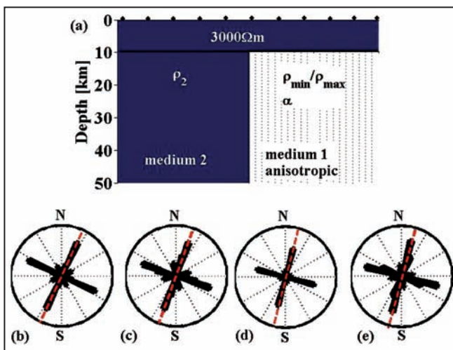
شکل ۲- مدل دوبعدی متشکل از یک گسل (محیط ۱ ناهمسانگرد با مقاومت ویژه‌های اصلی \rho_{min} = 10 \text{ m}\Omega / \rho_{max} = 3000 \text{ m}\Omega ، \alpha_s = 60^\circ و محیط ۲ همسانگرد) که توسط یک لایه مقاوم 3000 \text{ m}\Omega پوشیده شده است. (b تا e) نمودارهای گل‌سرخ نشان‌دهنده سوی امتداد برآورد شده برای باندهای دوره‌ای مختلف به ترتیب: 10000 \text{ s} ، 1000 \text{ s} ، 100 \text{ s} ، 10 \text{ s} . در بیشتر موارد این امتداد منطبق با روند ناهمسانگردی است.
