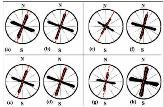
شکل ۵- سوهای استرایک وقتی مقاومت ویژه محیط ۲ 300 \Omega m ( \rho_p ) (شکل‌های a تا d) و 3 \Omega m (شکل‌های e تا h) باشد، برای باندهای دورهای مختلف (10 - 100000 s) ، (100 - 1000 s) ، (1000 - 10000 s) ، (10000 - 100000 s) .
