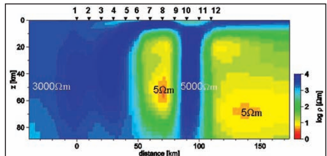
شکل ۶- مدل حاصل از وارون‌سازی داده‌ها پس از چرخش 60^\circ آنها. در صورت چرخش داده‌ها در سوی استرایک ناهمسانگردی، ماکروناهمسانگردی به‌صورت توالی بلوک‌های رساتا و مقاوم شیب‌سازی شده است.
