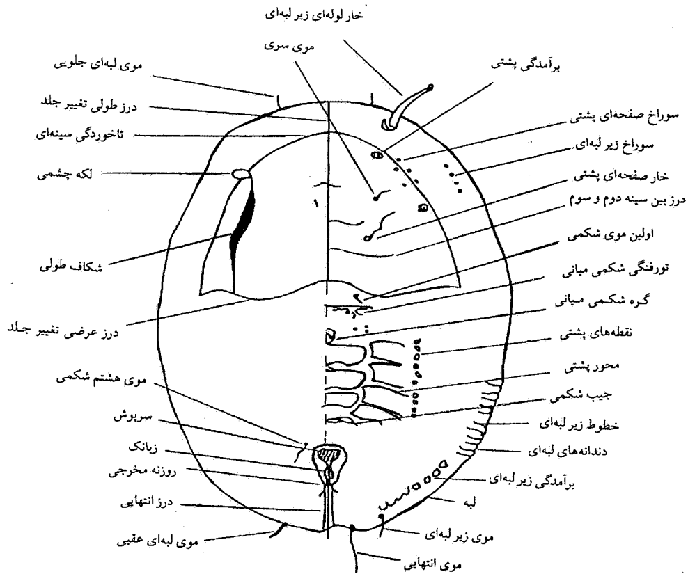
شکل ۵. سطح پشتی شفیره مگس سفید گلخانه (۲۰۰ برابر)
