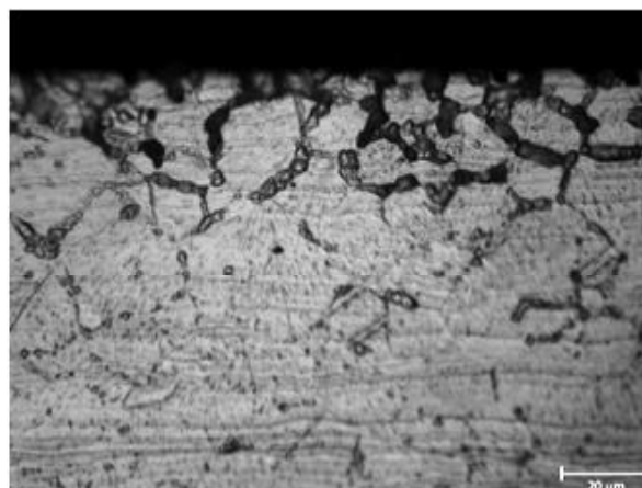
شکل ۳- ساختار میکروسکوپی عمق حساس شدگی آلیاژ ۳۱۶L عملیات حرارتی شده در ۸۰۰ °C به مدت ۳ ساعت، الکترو اچانت: اسید اگزالیک ۱۰ درصد
