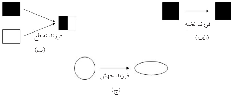
شکل ۳- نحوه تولید فرزندان در روش الگوریتم ژنتیک (الف) عملگر نخبه‌گرایی، (ب) عملگر تقاطع و (ج) عملگر جهش [۱۰]
