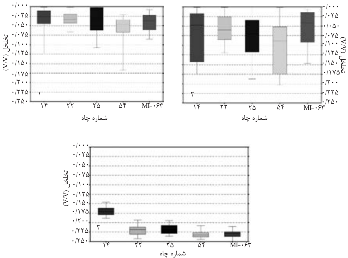
شکل ۸- میزان فراوانی تخلخل در رخساره‌های الکتریکی از رخساره شماره ۱ به سمت رخساره شماره ۳ در چاه‌های مطالعه شده
