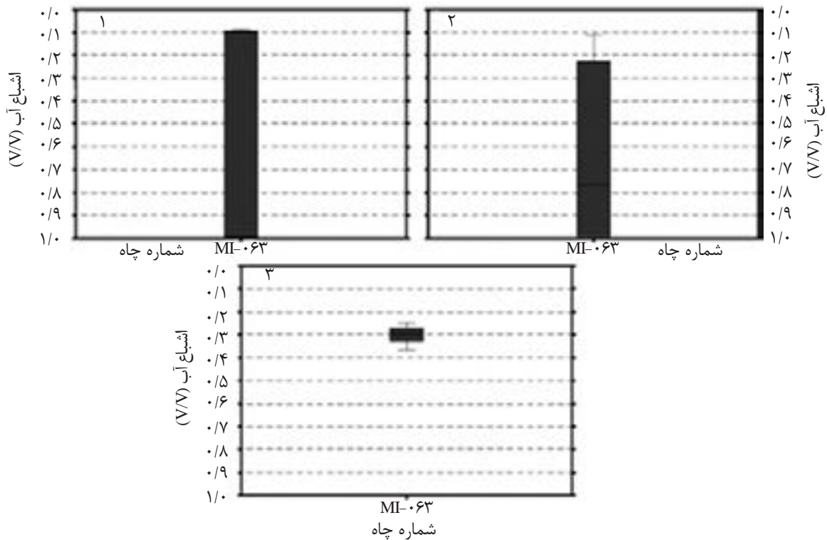
شکل ۹- روند کاهش درصد اشباع آب از رخساره ۱ به سمت رخساره ۳ در چاه ۶۳
