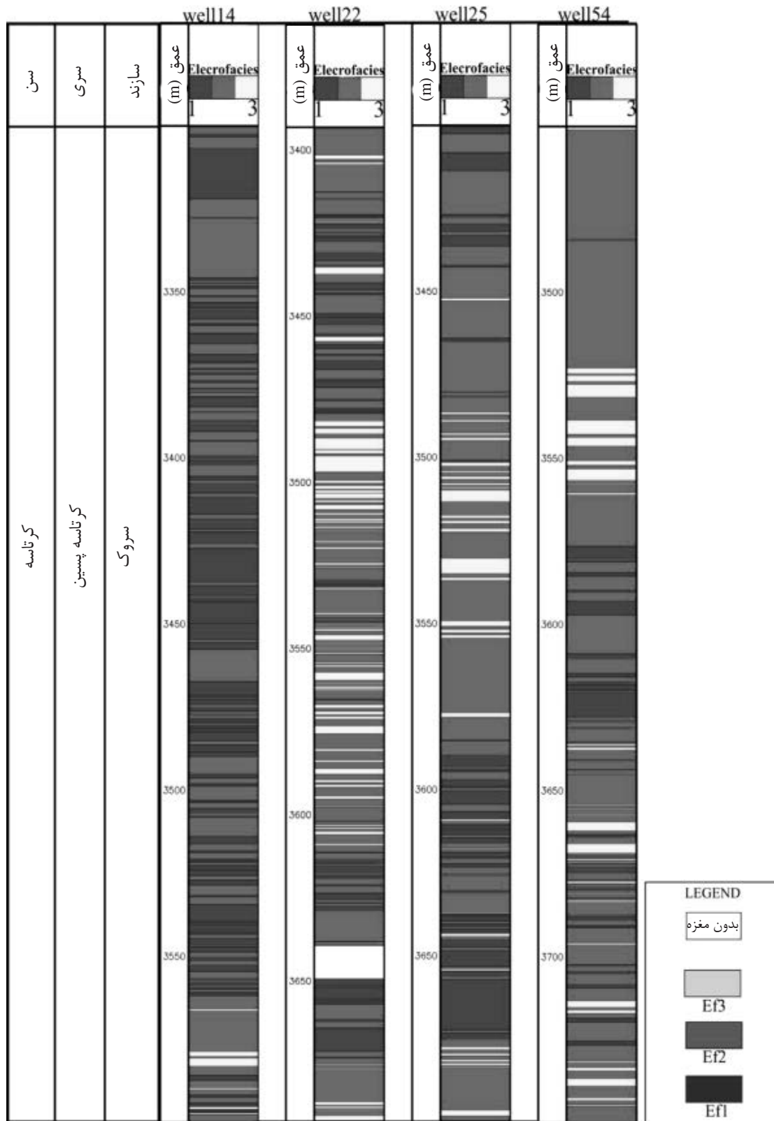
شکل ۱۱- مدل رخساره الکتریکی به دست آمده برای چاه‌های فاقد مغزه در میدان
