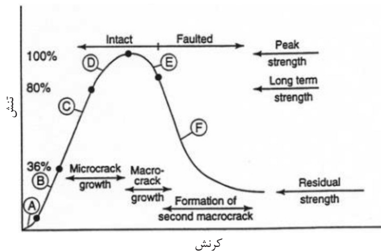
شکل ۸- نمودار تنش- کرنش [۱۲]
