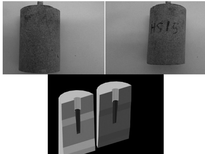
شکل ۴- شکست نمونه HS15
