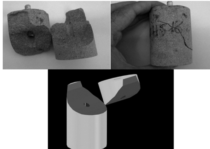
شکل ۵- شکست نمونه HS16
