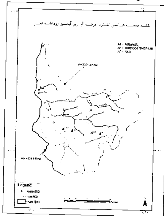
شکل ۱۵ تقسیم حوضه آبریز تجن به دو قسمت مجزا از محل آبراهه اصلی و نحوه محاسبه شاخص AF
