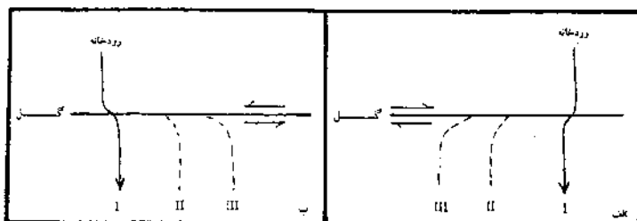
شکل ۷: تغییر شکل رودخانه به هنگام عبور از روی گسل های راستالغز (الف- راستگرد، ب- چپگرد): در مرحله
