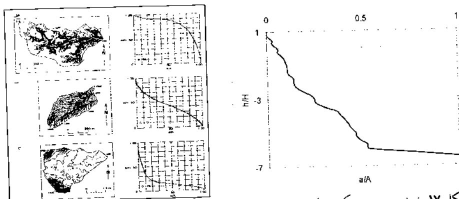
شکل ۱۷ منحنی هیسومتریک محاسبه شده رودخانه تجن شکل ۱۸ مثال هایی از انواع منحنی های فرازنا
