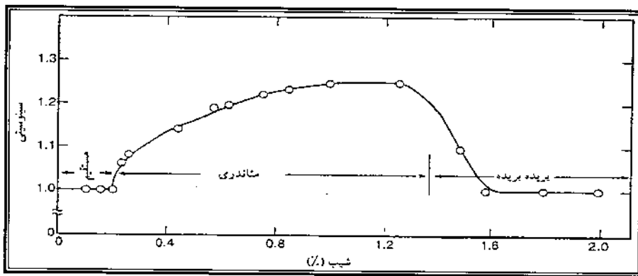
شکل ۱۱: رابطه میان شیب دره و مقدار سینوسیته کانال رودخانه در حین آزمایشات با دبی ثابت، بار رسوبی، قدرت رودخانه و مقدار سرعت آب با افزایش مقدار شیب، افزایش می یابد (سلیمانی، ۱۳۷۸، ۱۸).
