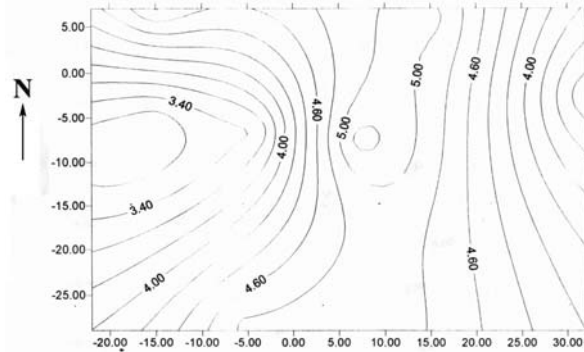
نمودار ۴- خطوط هم‌تراز آلایندة استیرین در خط استیرین در فصل پاییز
