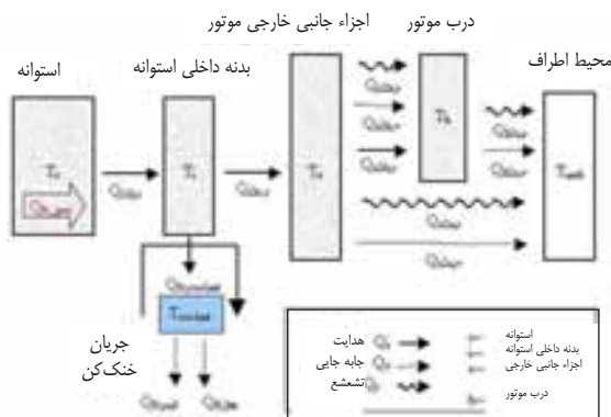
شکل ۳ الگوی حرارتی موتور
