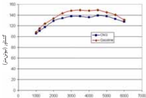
شکل ۴ منحنی گشتاور موتور ملی حالت گاز و بنزین سوزی (دور بر دقیقه)
