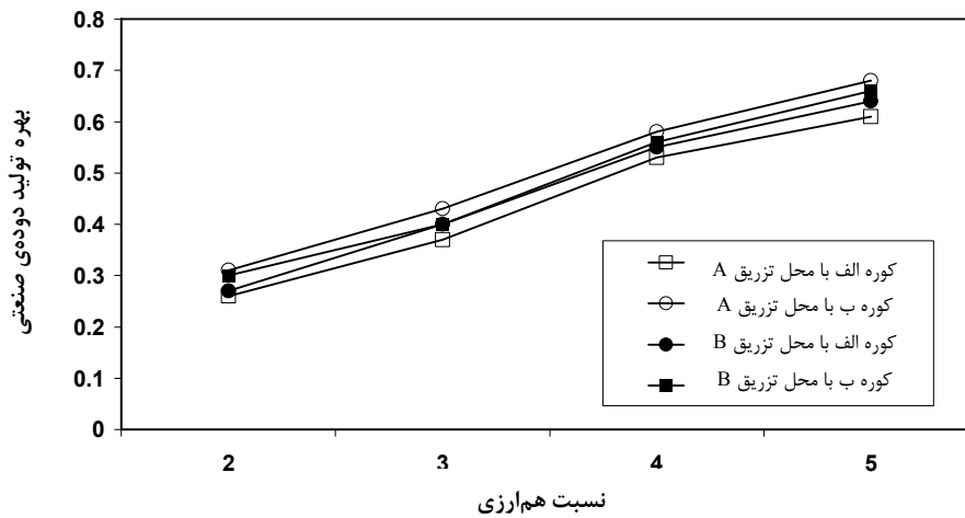
شکل ۸- بهره تولید سوخت استیلن در شرایط مختلف کوره
