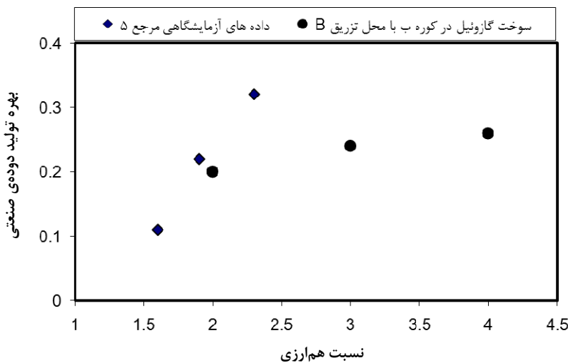
شکل ۷- مقایسه‌ی نتایج سوخت گازوییل با نتایج مرجع [۵]
