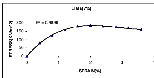
شکل ۶- منحنی تنش-کرنش حاصل از آزمایش
