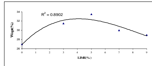
شکل ۱۲- تاثیر درصد وزنی آهک بر مقدار \omega_{opt}
