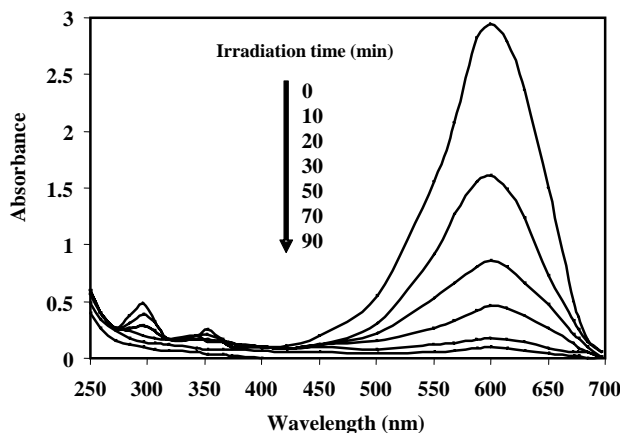
شکل ۲: تغییرات طیف‌های UV/Vis رنگزای بازیک آبی ۴۱ در فواصل زمانی مختلف تابش (غلظت رنگزا ۰/۱۱ mM، pH ۵/۵ و غلظت آب اکسیژنه ۷/۳ mM).
