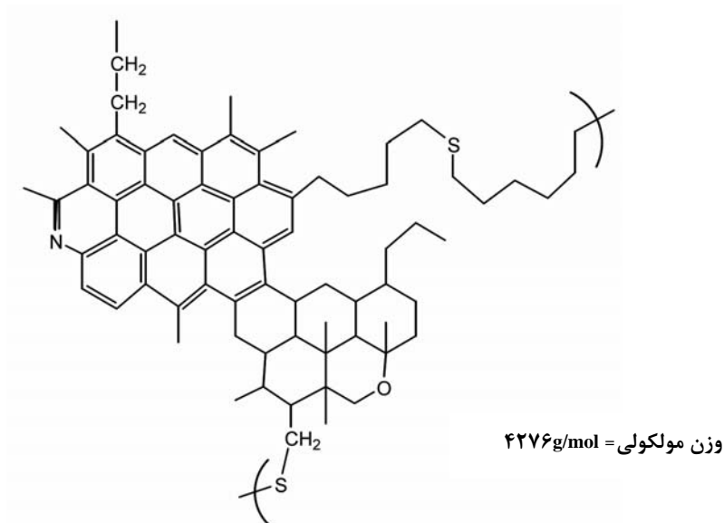
شکل ۲: یکی از ساختارهای فرضی آسفالتن‌ها [۸].
