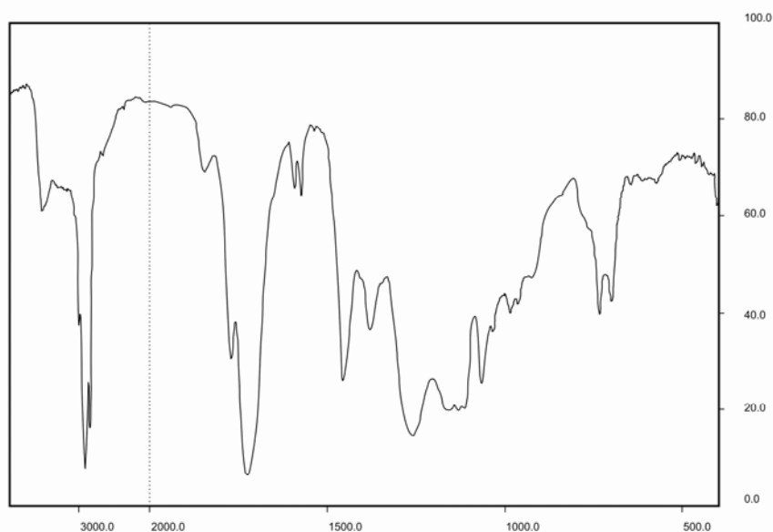
شکل ۹: طیف زیرقرمز رزین الکید آب پایه حاوی اسید چرب پیوند شده D5.
