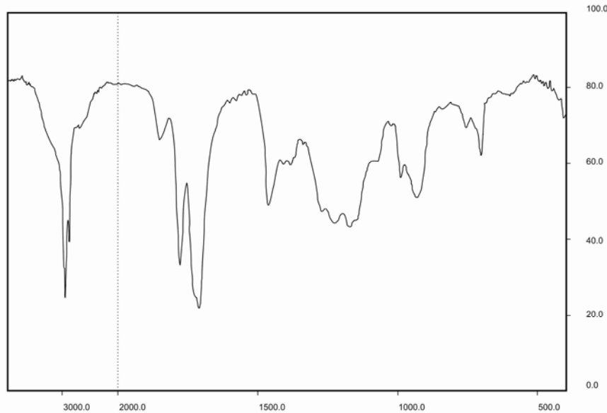
شکل ۵: طیف زیرقرمز اسید چرب پیوند شده C3.
