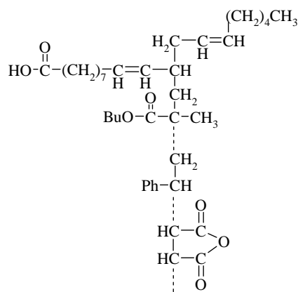
شکل ۲: ساختار شیمیایی تقریبی اسید چرب سویای پیوند شده.
