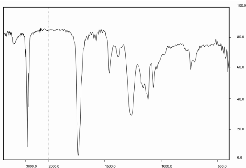
شکل ۷: طیف زیر قرمز رزین الکید A3.
