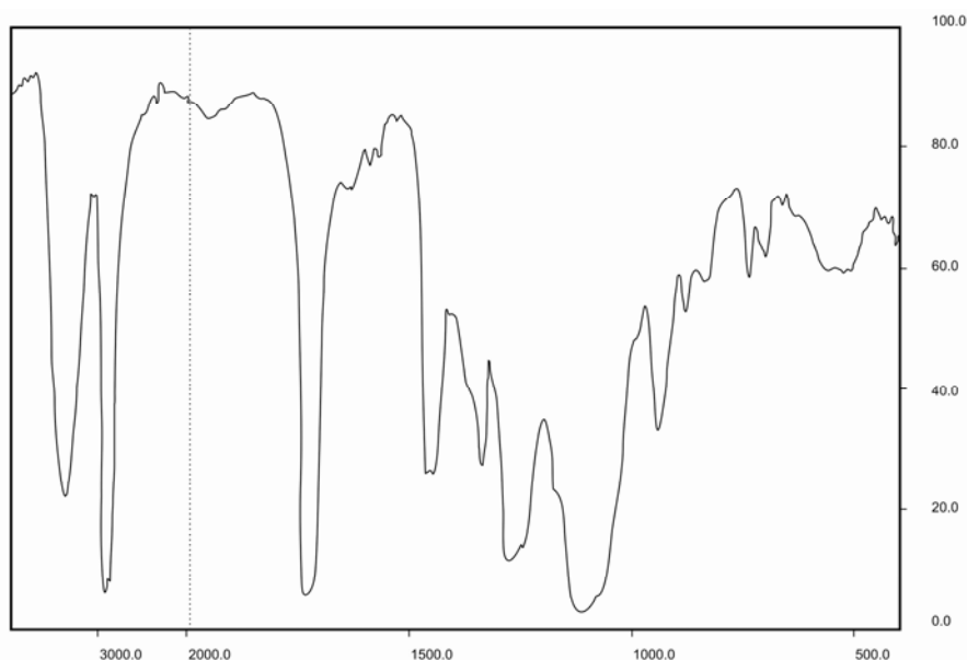
شکل ۱۱: طیف زیرقرمز رزین الکید هیبرید ترکیبی E2.
