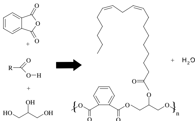
شکل ۱: واکنش تولید و ساختار رزین آلکید.
