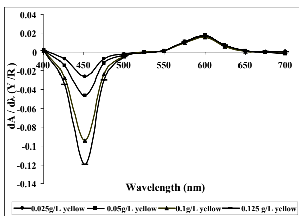
شکل ۸: مشتق طیف‌های نسبی مخلوط‌های زرد و قرمز (۰/۰۵ g/L قرمز به عنوان استاندارد).
