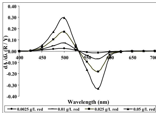
شکل ۷: مشتق طیف‌های نسبی مخلوط‌های زرد و قرمز (۰/۰۵ g/L زرد به عنوان استاندارد).
