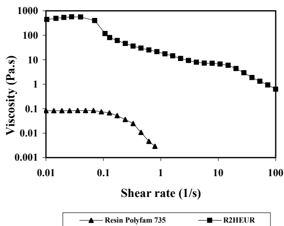
شکل ۵: مقایسه رفتار گرانشی بر علیه سرعت برشی رزین پلی‌فام ۷۳۵ و نمونه R2HEUR (رزین حاوی ۱,۱۵٪ غلظت‌دهنده).
