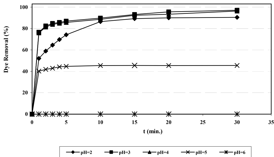
شکل ۲: اثر pH بر میزان و سرعت رنگبری در 0.3 \text{ mM} ، \text{Fe}(\text{II}) ، در 3 \text{ mM} ، \text{H}_2\text{O}_2 ، 100 \text{ mg/l} ، [\text{RR120}]_0 ، دمای محیط و بدون هم‌زدن.
