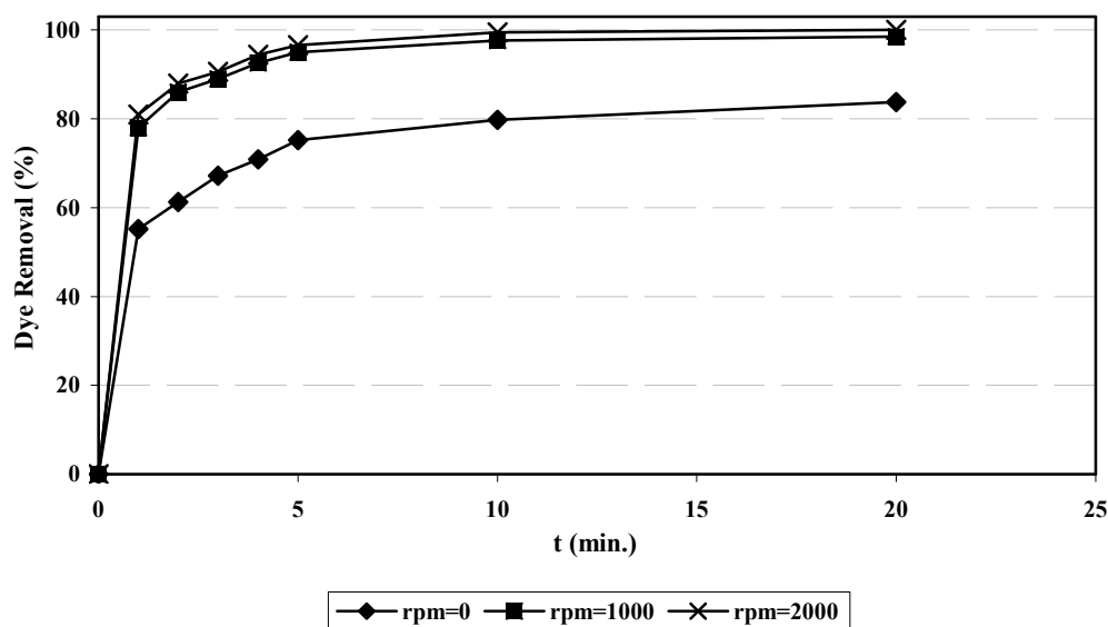
شکل ۸: اثر دور هم‌زدن در pH=۳ و [Fe 2+ ] 0 =۰,۳ mM و [H 2 O 2 ] 0 =۳ mM بر رنگبری از محلول ۱۰۰ ppm رنگزای RR120.
