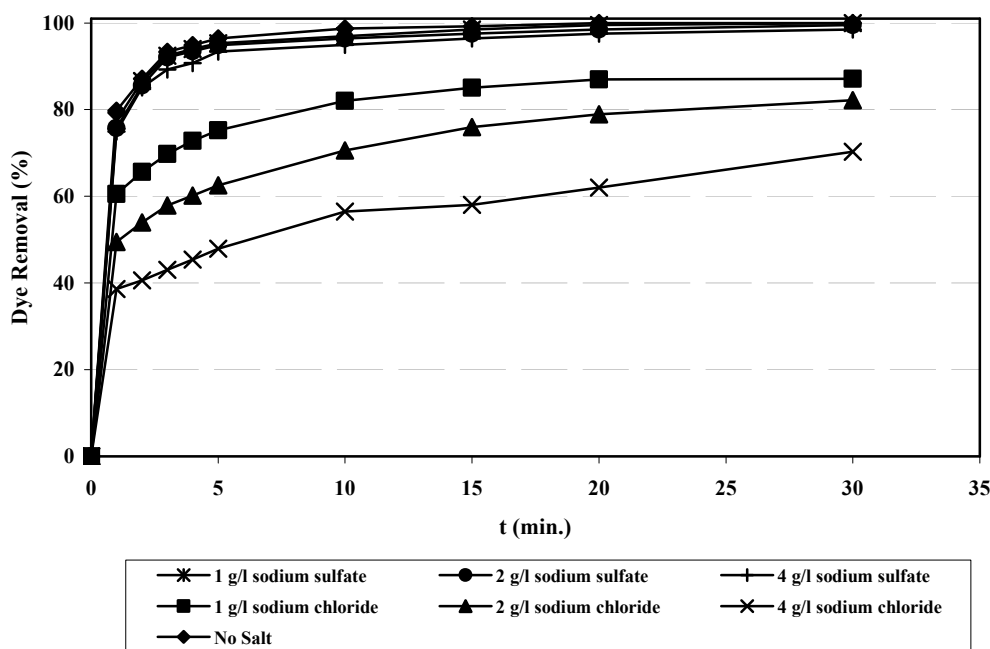
شکل ۷: اثر غلظت الکترولیت NaCl و Na 2 SO 4 بر میزان رنگبری در pH=۳ و [Fe 2+ ] 0 =۰,۳ mM و [H 2 O 2 ] 0 =۳ mM.
