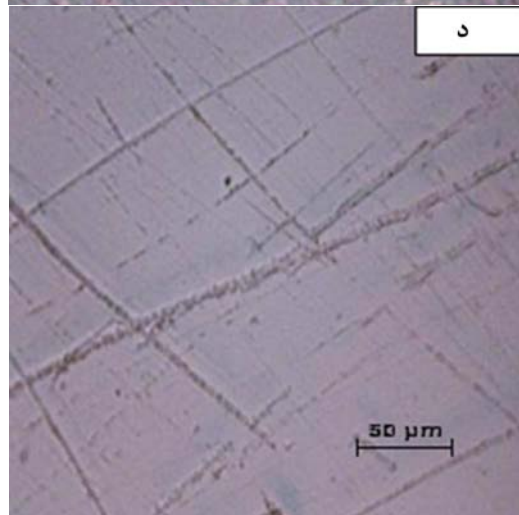
شکل ۵: تصاویر میکروسکوپ نوری از سطح ساییده شده: الف) نمونه T_{0.25}^{0.25} ، ب) پلی‌کربنات، ج) نمونه T_4^1 ، د) نمونه T_1^1 .
