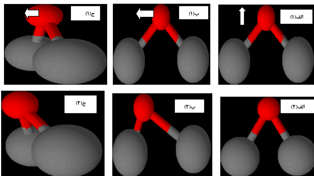
شکل ۳: شکل شماتیک حرکت نوسانی اتم اکسیژن نسبت به اتم‌های سیلیکون. الف) کشش متقارن اتم اکسیژن در راستای نیمساز زاویه Si-O-Si، ب) کشش نامتقارن اتم اکسیژن موازی با خط فرضی اتصال دهنده اتم‌های سیلیکون، ج) تحرک rocking عمود بر صفحه Si-O-Si.
