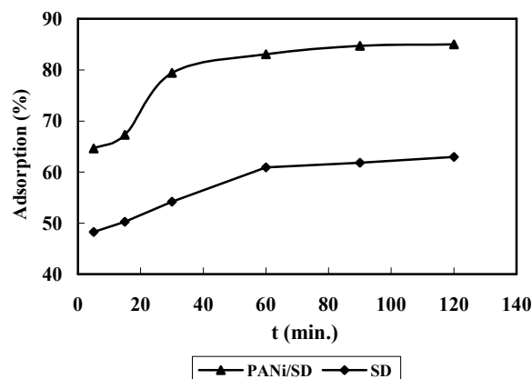
شکل ۵: تأثیر زمان تماس بر میزان حذف CR با PANi/SD، SD (غلظت اولیه: ۵۰ ppm، مقدار جاذب ۰.۶۰ g، زمان تماس ۵-۱۲۰ دقیقه، pH=۶).
