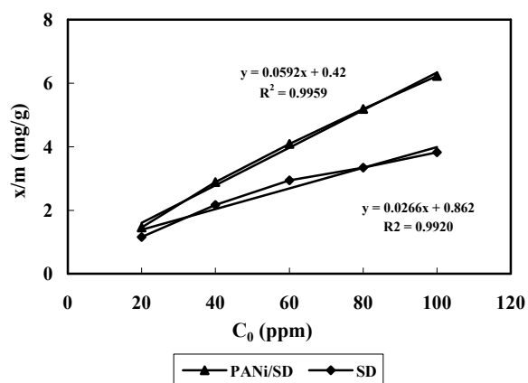
شکل ۳: تأثیر غلظت اولیه CR بر روی میزان حذف توسط PANi/SD، SD (غلظت اولیه: ۱۰۰-۲۰ ppm، مقدار جذب ۰٫۶۰ g، زمان تماس ۶۰ دقیقه، pH = 6 ).
