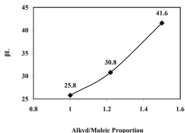
شکل ۱۰: منحنی شدت فلورسانس رزین آلکید بلند روغن و ورنی مالئیک حاوی ۰,۵ درصد ورنی رنگزای D.Y.۲۳۲ برحسب درصد اختلاط دو رزین (روش محاسبه اختلاف انعکاس دو منحنی انعکاسی در طول موج بیشینه نشر می باشد).
