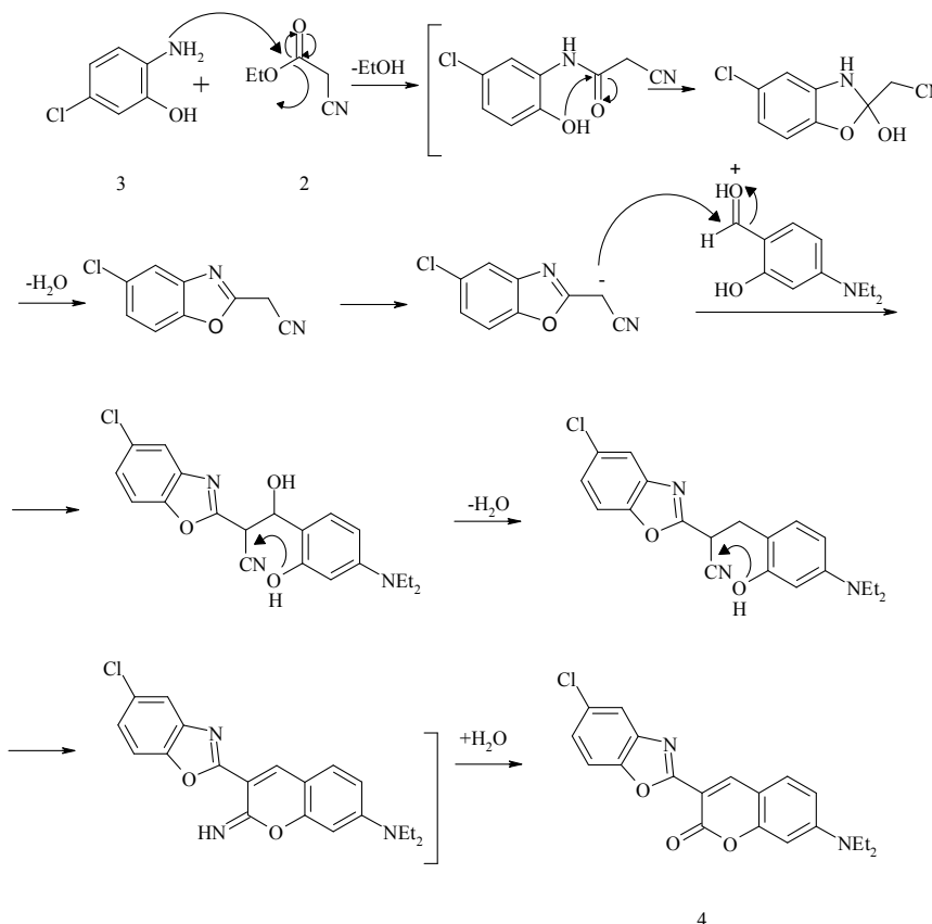
شمای ۲: سازوکار تشکیل ترکیب ۴.
