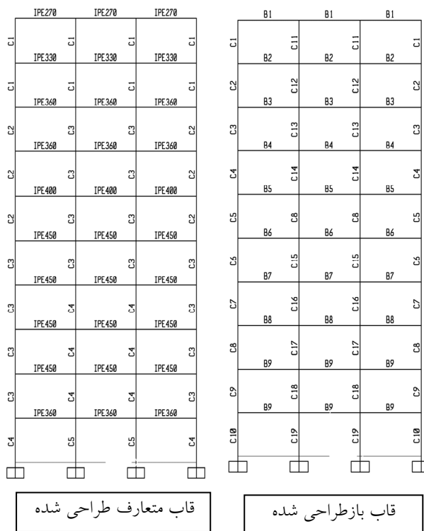
شکل (۵): ابعاد اعضای طراحی شده دو قاب خمشی ۱۰ طبقه به روش انرژی (قاب بازطراحی شده) و استاتیکی معادل (قاب متعارف طراحی شده)
