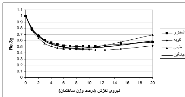
شکل (۱۲): فاکتور کاهش انرژی مانده ساختمان هشت طبقه تحت زلزله‌های 0.3g
