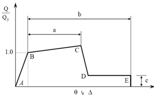
شکل (۲): منحنی نیرو-تغییر شکل تعمیم یافته برای اعضای فولادی [21] و [22]
