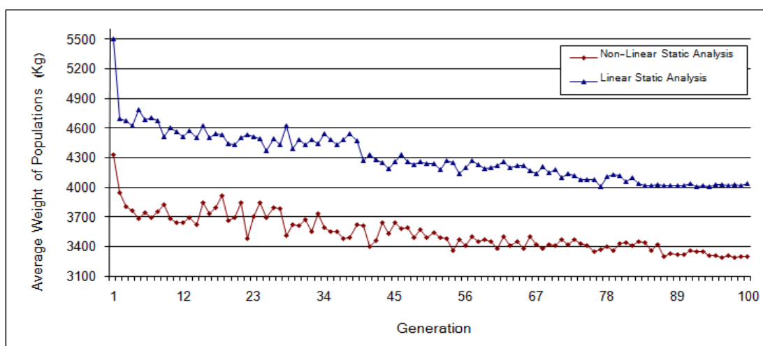
شکل (۷): مقایسه تاریخچه تغییرات وزن در قاب شش طبقه یک دهانه با اتصالات نیم صلب (قاب ۴) تحت تحلیل خطی و غیر خطی
