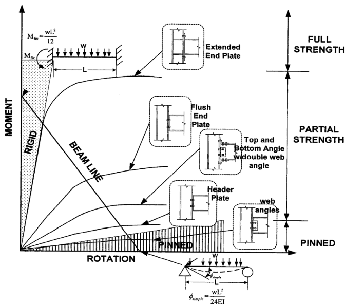
شکل (۱): رابطه لنگر-دوران اتصال های فولادی [۲۰].
