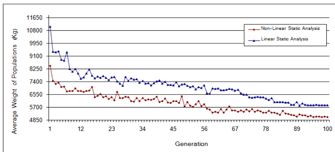
شکل (۸): مقایسه تاریخچه تغییرات وزن در قاب نه طبقه یک دهانه با اتصالات نیم صلب (قاب ۷) تحت تحلیل خطی و غیر خطی
