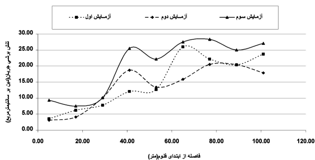
شکل ۳- نمودار تغییرات تنش برشی جریان در طول بستر فلوم در آزمایش های گوناگون
