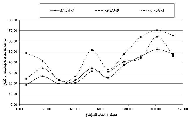
شکل ۲- نمودار تغییرات میانگین سرعت جریان در طول بستر فلوم در آزمایش های گوناگون
