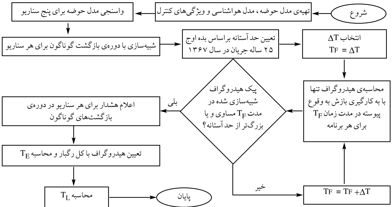
شکل ۲ - فلوچارت محاسبه ی زمان پیش هشدار با استفاده از مدل HEC-HMS
