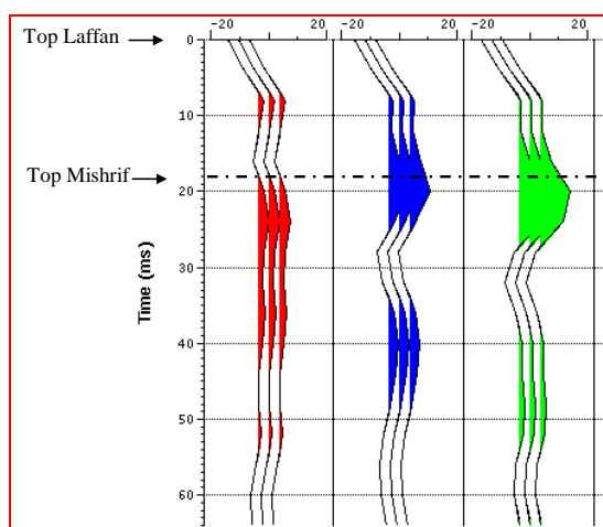
شکل ۱۰. تریس های میانگین مربوط به روش با نظارت با سه رخساره.
