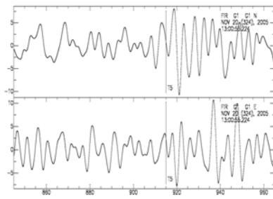
شکل ۲. سمت چپ-بالا) لرزه‌نگاشت سه مؤلفه رویداد دورلرز ۳ دسامبر ۲۰۰۵ با بزرگی ۵٫۸ که در ایستگاه لرزه‌نگاری کاوش (IIES) ثبت شده است ( \Delta = 83.0^\circ و BAZ = 80.1^\circ )، پایین) مؤلفه‌های افقی لرزه‌نگاشت بالا) فاز SKS با خط عمودی نشان داده شده است (سمت راست-بالا) لرزه‌نگاشت سه مؤلفه رویداد دورلرز ۲۰ نوامبر ۲۰۰۵ با بزرگی ۶٫۲ که در ایستگاه لرزه‌نگاری فیروزکوه (IGTU) ثبت شده است ( \Delta = 85.4^\circ و BAZ = 20.9^\circ )، پایین) مؤلفه‌های افقی لرزه‌نگاشت بالا) فاز SKS با خط عمودی نشان داده شده است.
