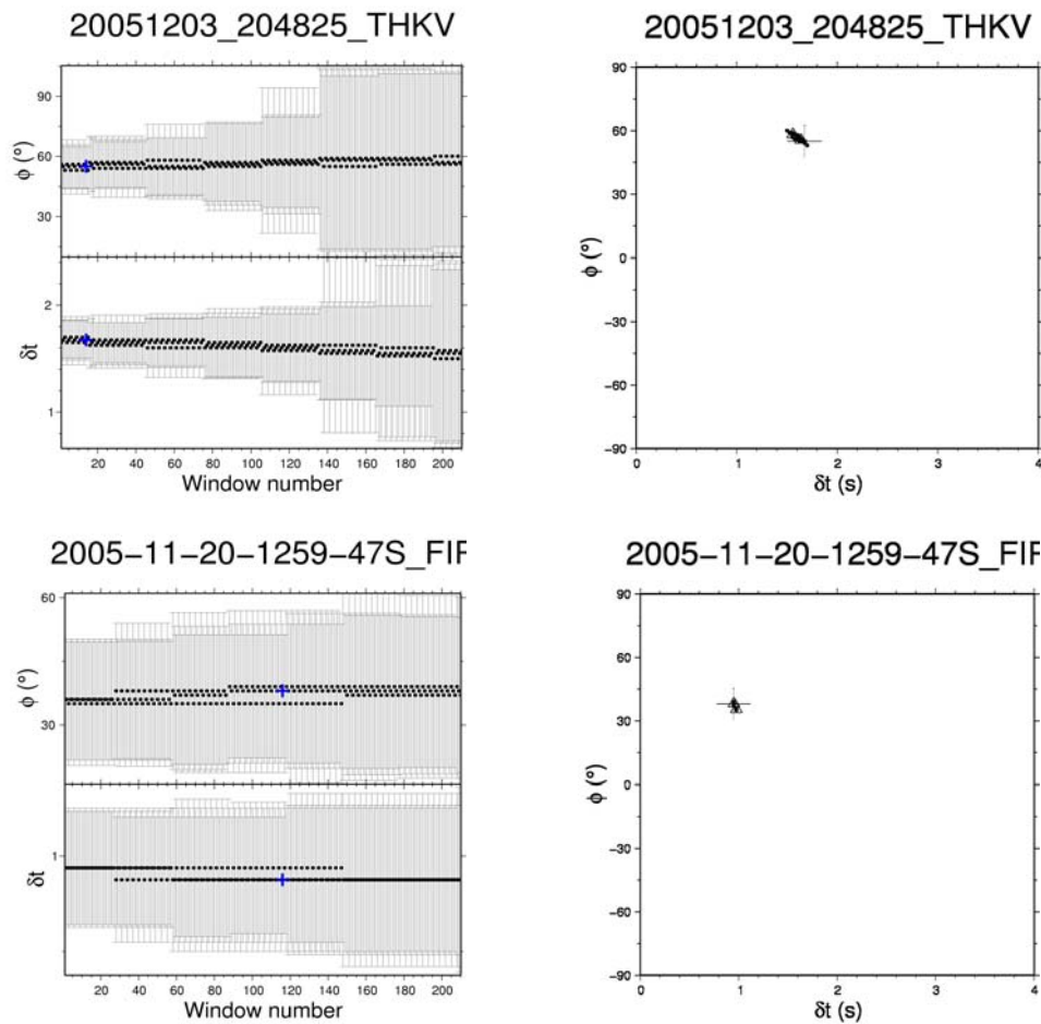
شکل ۶. (چپ) رسم خطای محاسبه \delta t و \varphi برحسب شماره پنجره، کم خطاترین \delta t و \varphi با + مشخص شده است و (راست) نمودار جواب‌های روش تحلیل خوشه‌ای به منظور دستیابی به \delta t و \varphi بهینه، بهترین جواب با به‌علاوه مشخص شده است (بالا) مربوط به رویداد دورلرز ۳ دسامبر ۲۰۰۵ با بزرگی ۵٫۸ که در ایستگاه لرزه‌نگاری کاوش (IIEES) ثبت شده است ( \delta t = 1.68 \text{ sec.} , \varphi = 55^\circ ). (پایین) مربوط به رویداد دورلرز ۲۰ نوامبر ۲۰۰۵ با بزرگی ۶٫۲ که در ایستگاه لرزه‌نگاری فیروزکوه (IGTU) ثبت شده است ( \delta t = 0.95 \text{ sec.} , \varphi = 38^\circ ).
