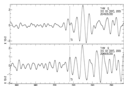
شکل ۲. سمت چپ-بالا) لرزه‌نگاشت سه مؤلفه رویداد دورلرز ۳ دسامبر ۲۰۰۵ با بزرگی ۵٫۸ که در ایستگاه لرزه‌نگاری کاوش (IIES) ثبت شده است ( \Delta = 83.0^\circ و BAZ = 80.1^\circ )، پایین) مؤلفه‌های افقی لرزه‌نگاشت بالا) فاز SKS با خط عمودی نشان داده شده است (سمت راست-بالا) لرزه‌نگاشت سه مؤلفه رویداد دورلرز ۲۰ نوامبر ۲۰۰۵ با بزرگی ۶٫۲ که در ایستگاه لرزه‌نگاری فیروزکوه (IGTU) ثبت شده است ( \Delta = 85.4^\circ و BAZ = 20.9^\circ )، پایین) مؤلفه‌های افقی لرزه‌نگاشت بالا) فاز SKS با خط عمودی نشان داده شده است.
