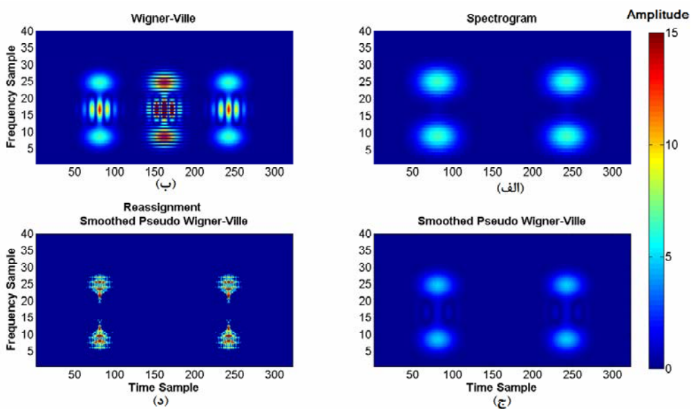
شکل ۲. توزیع زمان-فرکانس سیگنال شکل ۱ با استفاده از چهار روش (الف) طیف‌نگاشت، (ب) توزیع ویگنر-وایل، (ج) توزیع ویگنر-وایل نمای هموار شده و (د) شکل بازچینی شده توزیع ویگنر-وایل نمای هموار شده.
