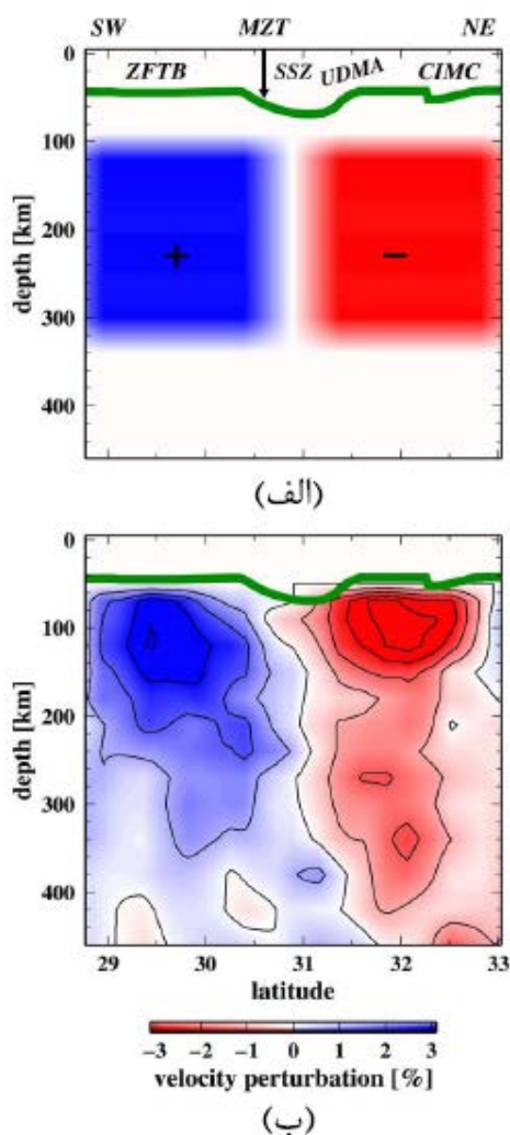
شکل ۷. (الف) مقطع عرضی ساختار سرعت فرضی برای نیمرخ زاگرس. بی‌هنجاری آبی‌رنگ ساختار سرعت با +3\% و بی‌هنجاری سرخ‌رنگ ساختار سرعت با -3\% را نسبت به مدل یک‌بندی IASP91 نشان می‌دهد. (ب) مدل بازیابی‌شده از ساختار فرضی پس از تکرار سوم.
