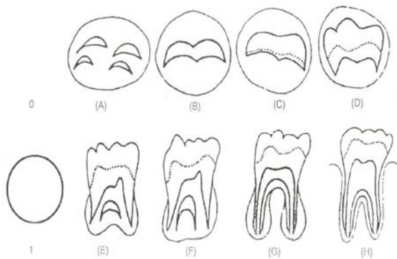
شکل ۱. مراحل A تا H تکامل مولر سوم در روش دمرجیان
