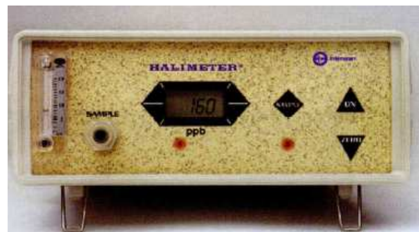
شکل ۱. دستگاه Halimeter [۴]
