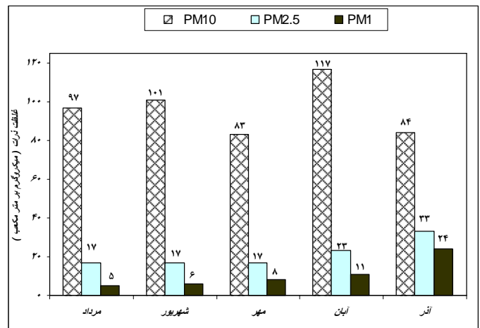
نمودار شماره ۲: مقایسه میانگین مقادیر PM_{10} ، PM_{2.5} ، PM_1 در ماه‌های تابستان و پاییز ۱۳۸۶
