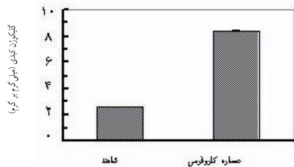
نمودار 3: اثر تجویز عصاره کلروفومی به میزان 3 میلی‌گرم به ازای هر کیلوگرم روی میزان گلیکوژن کبدی
