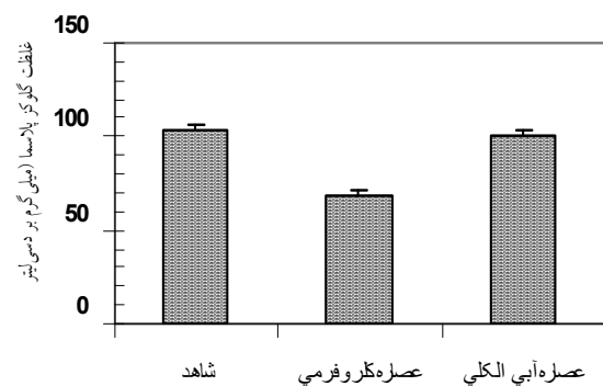
نمودار 2: اثر تجویز عصاره‌های آبی-الکلی و کلروفومی به مقدار 3 میلی‌گرم به ازای هر کیلوگرم وزن بدن بر غلظت گلوکز پلاسمای ناشتا
