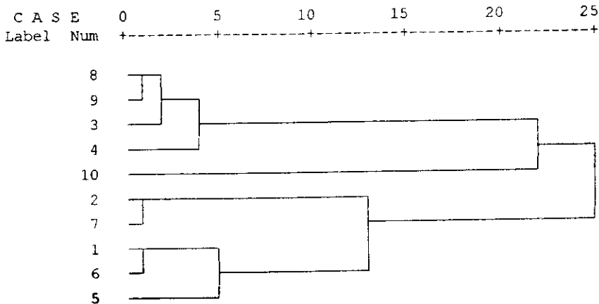
نمودار ۴: دارنگاره (Dendrogram) حاصل از آنالیز دسته بندی خوشه ای (Cluster Analysis) بین ایستگاههای نمونه برداری با توجه به تشابه آنها از نظر فراوانی میوبنتوزها و خصوصیات رسوبات بستر در خورهای شمالی استان بوشهر (سال ۸۰ - ۱۳۷۹)
