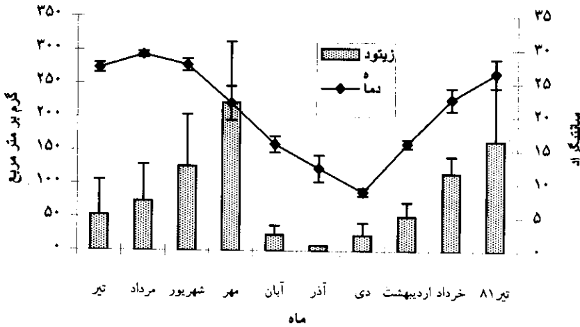
نمودار ۳: تغییرات زیتوده شانه‌دار و دمای آب در دریای خزر سال ۸۱-۱۳۸۰
