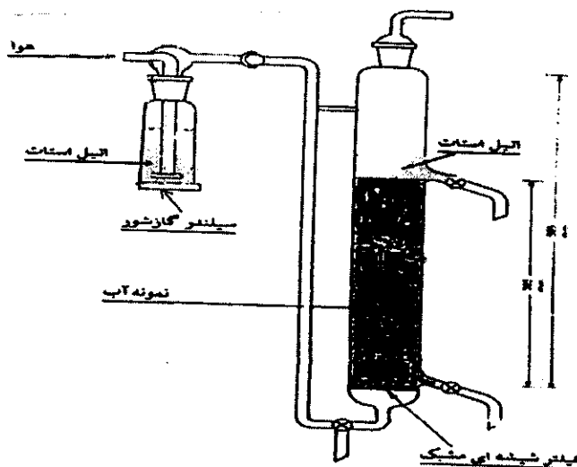
شکل ۲: دستگاه سابلیشن
