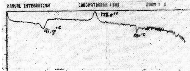
نمودار ۷: طیف DSC مستر بیج (زرد کم رنگ) حاوی عامل شبکه کننده
