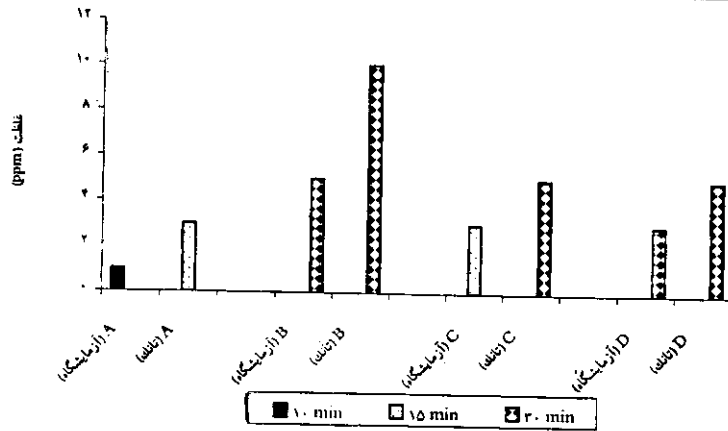
نمودار ۱: مقایسه حداقل غلظت / زمان موثر ضد عفونی کننده‌های کلرهگزیدین (A)، پرمنگنات پتاسیم (B)، هیپوکلریت سدیم (C) و ستریمایدت (D) در شرایط آزمایشگاه و تانک‌های پرورش بر باکتری استرپتوکوکوس اینیایی جدا شده در فاصله سالهای ۱۳۸۱-۱۳۸۳
