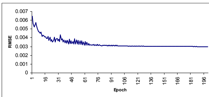
شکل ۳- مقدار RMSE در تکرارهای آموزش شبکه‌های عصبی فازی شرکت پتروشیمی آبادان
