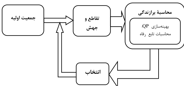
شکل ۴: روند اجرای الگوریتم ژنتیک پیشنهادی
