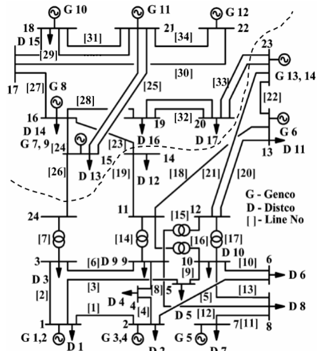
شکل ۵: شبکه ۲۴ بسته IEEE-RTS
