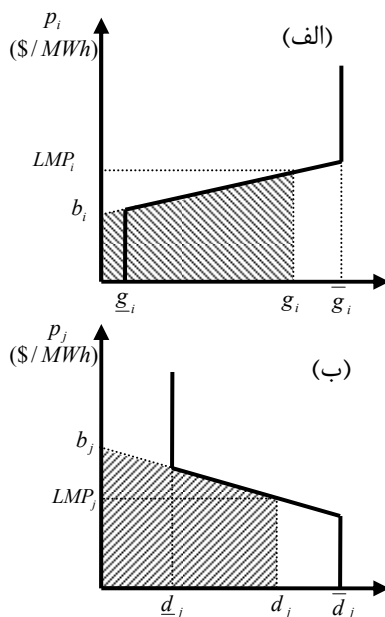
شکل ۱: منحنی‌های پیشنهاد قیمت برای (الف) تولیدکنندگان (ب) مصرف‌کنندگان
