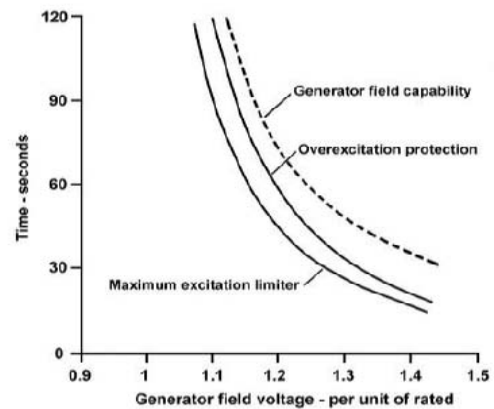
شکل ۲- منحنی اضافه بار - زمان برای تحریک ژنراتور
