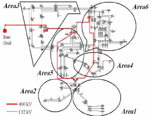
شکل ۱۲- تقسیم بندی شبکه خراسان به ۶ ناحیه بار در روش VCI
