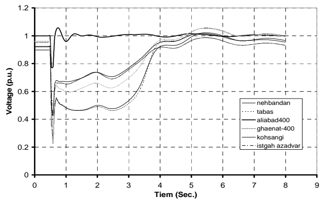
شکل ۸- ولتاژ برخی از باسهای خراسان در حادثه شماره ۲
