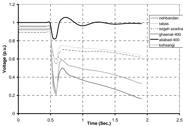
شکل ۷- ولتاژ برخی از باسهای خراسان در حادثه شماره ۱
