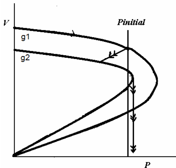
شکل ۶- فروپاشی ولتاژ گذرا در یک اغتشاش بزرگ نوعی
