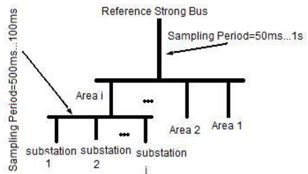
شکل ۱۱- ساختار مخابراتی پیشنهادی در روش VCI
