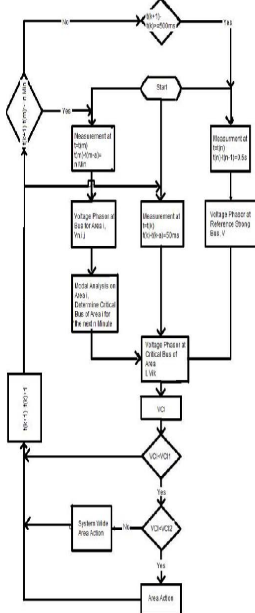
شکل ۱۳- فلوچارت الگوریتم VCI
