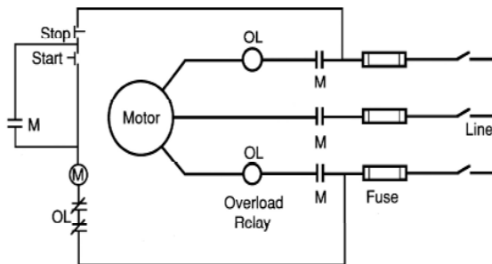
شکل ۵- یک نمونه مدار اتصال یک موتور القایی به شبکه از طریق کنتاکتور
