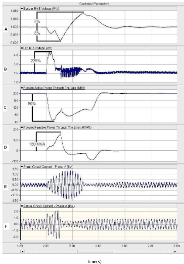
شکل (۸): نتایج شبیه سازی روش جدید در زمان وقوع خطا برای مدار نمونه ۲: (A) ولتاژ باس خروجی ترانسفورماتور (pu) ولتاژ DC خازن (B) توان اکتیو عبوری از خط انتقال (MW) (C) توان راکتیو عبوری از خط انتقال (MVAR) (E) جریان شاخه موازی UPFC (F) جریان خط انتقال
