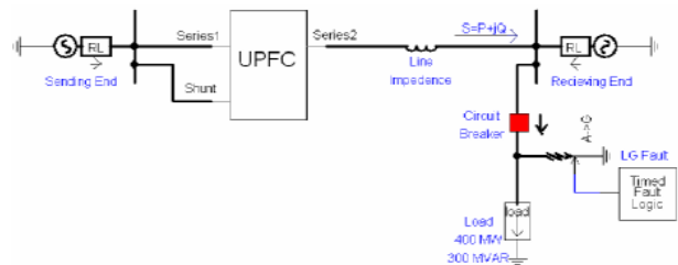
شکل (۱): نحوه اتصال UPFC به شبکه
