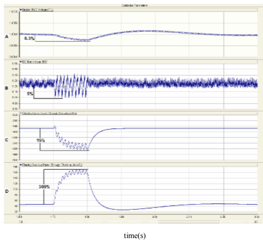
شکل (۶): نتایج شبیه‌سازی روش قدیم ۱ در زمان وقوع خطا برای مدار نمونه (A: ولتاژ باس (pu) Sending End (B) ولتاژ DC خازن (kV) توان اکتیو عبوری از خط انتقال (MW) (D) توان راکتیو عبوری از خط انتقال (MVAR))
