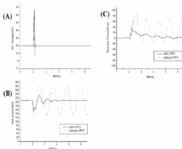
شکل (۹): نتایج شبیه‌سازی روش قدیم ۲ در زمان وقوع خطا برای مدار نمونه ۲: (A) ولتاژ DC خازن (kV) و توان اکتیو عبوری از خط انتقال (MW) (C) توان راکتیو عبوری از خط انتقال (MVAR)
