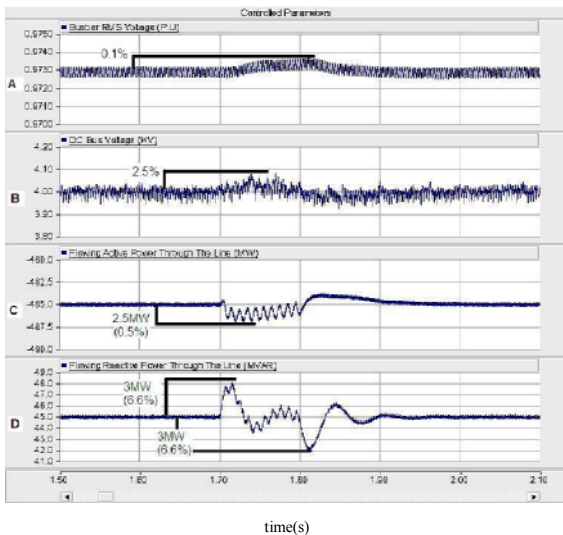
شکل (۵): نتایج شبیه‌سازی روش جدید در زمان وقوع خطا برای مدار نمونه (A: ولتاژ باس (pu) Sending End (B) ولتاژ DC خازن (kV) توان اکتیو عبوری از خط انتقال (MW) (D) توان راکتیو عبوری از خط انتقال (MVAR))
