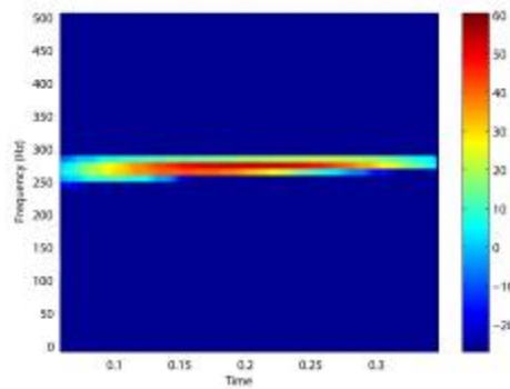
شکل (8): نمایش زمان - فرکانس تبدیل چیرپلت از خودروی متحرک
