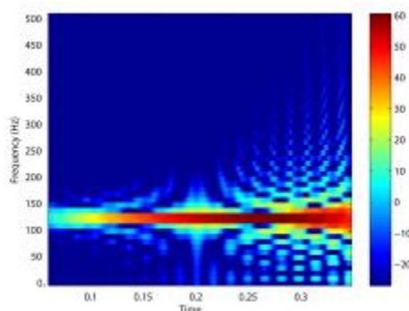
شکل (6): نمایش زمان - فرکانس تبدیل چیرپلت از انسان متحرک
