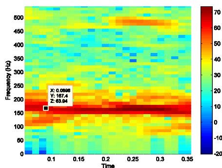
شکل (4): اسپکتروگرام به دست آمده از حیوان متحرک
