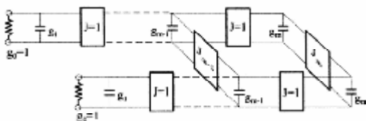
شکل (3): مدار معادل فیلتر پایین گذر با یک جفت صفر انتقال محدود [7]
