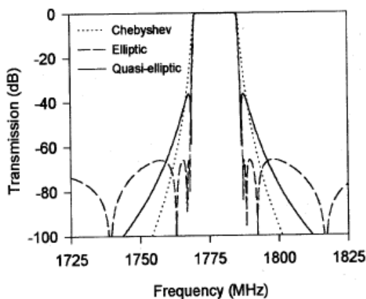
شکل (2): پاسخ فرکانسیهای سه نوع فیلتر میانگذر [6]
