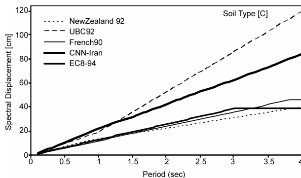
شکل ۲- طیف تغییرمکان ایران برای خاک نوع دو و مقایسه آن با طیفهای آیین‌نامه‌ای دیگر.
