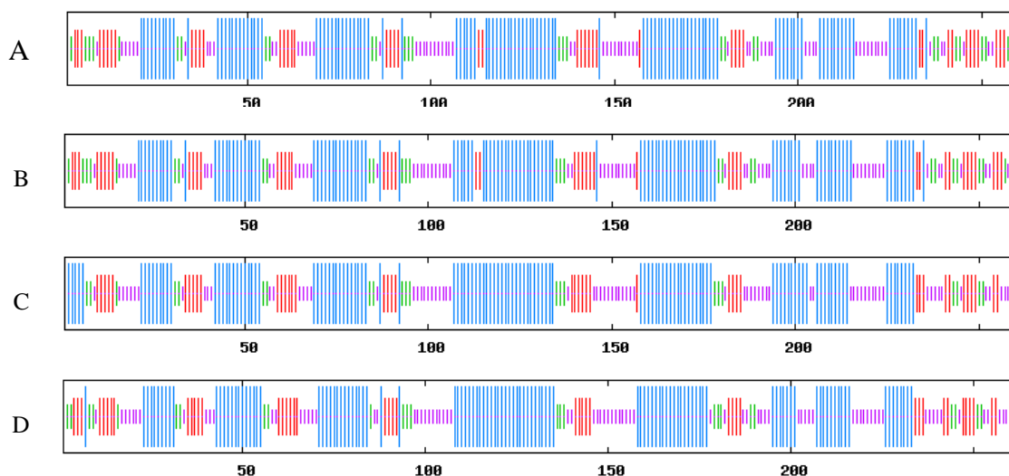
شکل ۴: ساختار دوم پروتئین TR-II گیاه هدف با استفاده از برنامه SOPMA و مقایسه آن با توالی پروتئینی در سه گیاه دیگر: Hyoscyamus niger (گیاه بنگدانه هدف)، Hyoscyamus niger (گیاه بنگدانه موجود در NBI)، Datura stramonium (C) و Solanum tuberosum (D) و مارپیچ \alpha (خطوط آبی)، صفحه \beta (خطوط قرمز)، پیچ \beta (خطوط سبز) و مارپیچ تصادفی (خطوط بنفش).
