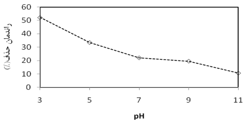
شکل ۳: تأثیر تغییرات pH بر روی کارایی حذف رنگ (غلظت اولیه رنگ ۴۰ mg/l، مقدار اولیه جاذب ۵۰/۵ gr/50cc)
