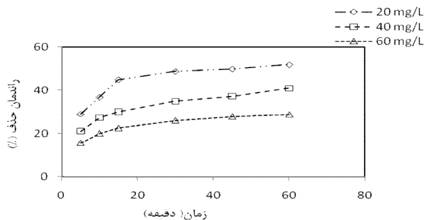
شکل ۲: تأثیر زمان تماس بر روی کارایی حذف رنگ (pH=۳، و مقدار اولیه جاذب ۵۰/۵ gr/50CC)
