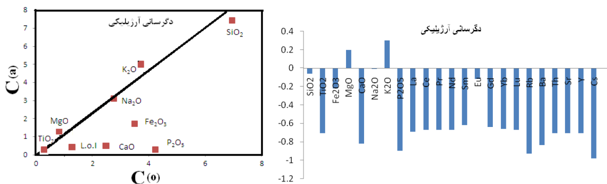
شکل ۶- نمودار تغییرات اکسیدهای اصلی به همراه نمودار تهی‌شدگی-غنی‌شدگی برای پهنه دگرسانی آرژیلیک
