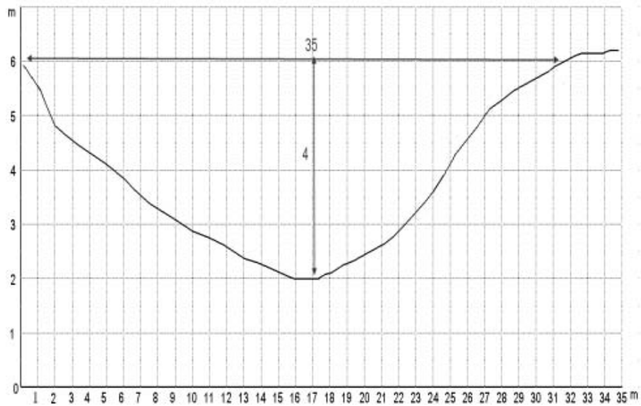
شکل شماره‌ی ۶- پروفیل عرضی خندق شماره دو، واحد به متر
