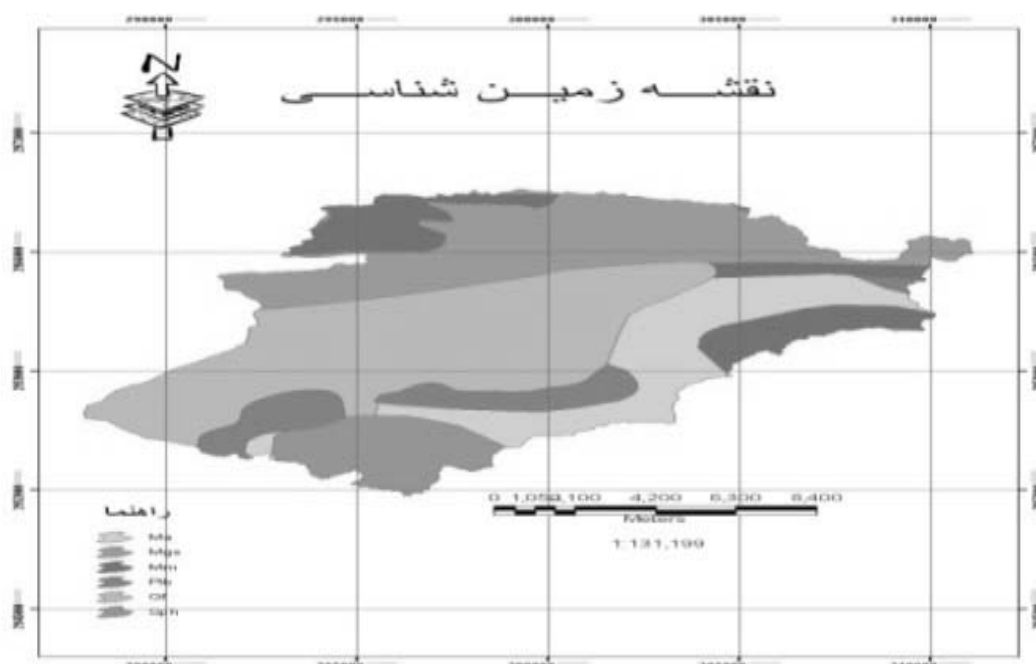
شکل شماره ۲- زمین شناسی حوضه‌ی آبخیز گزیر
