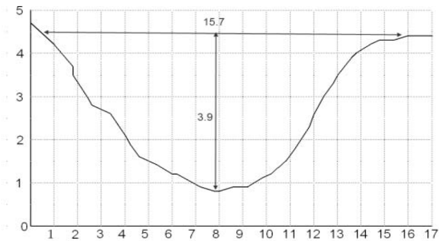
شکل شماره‌ی ۸- پروفیل عرضی خندق شماره سه، واحد به متر
